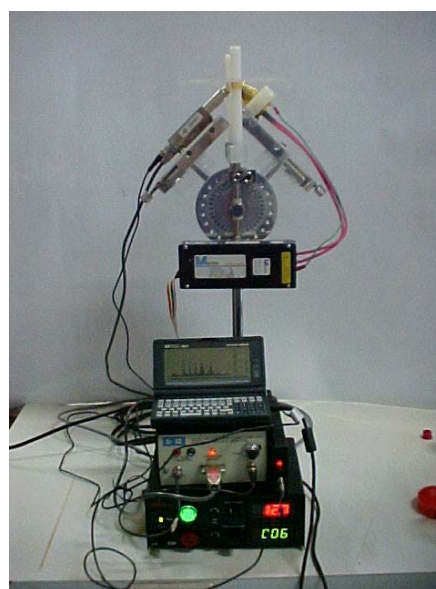
Fig.2 O sistema portátil de EDXRF com detector não-criogênico de Si-PIN para uso com mini tubo de raios X com anodo de Ag.
