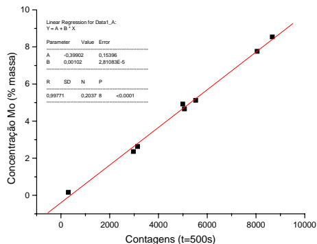
Fig.4 Correlação entre contagens e quantidade de Mo nos padrões de aço medidos por EDXRF portátil.
