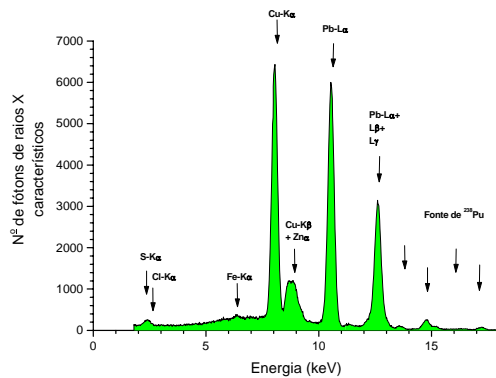
Fig. 8 Espectro de Raios X de uma região com corrosão cinza Edan A.
