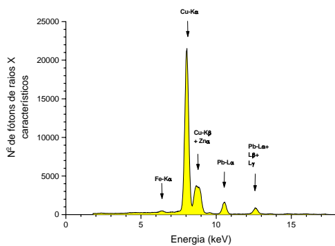
Fig. 7 Espectro de Raios X de uma região sem corrosão do Edan A.
