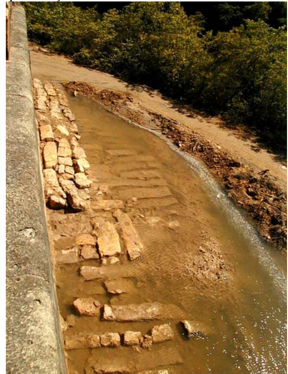
Figura 10 - estrutura de defesa contra as águas do riacho que contorna o Forte.
